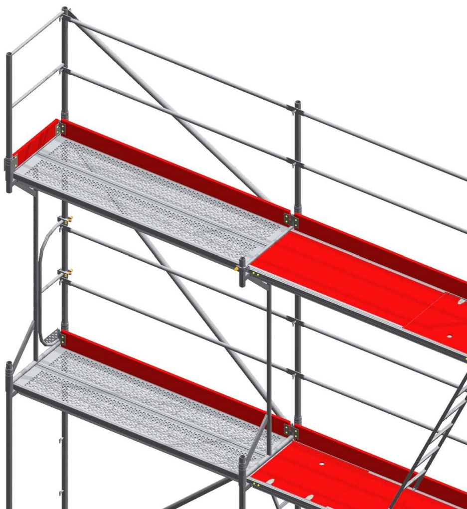
Rys. 1. Sposób zabudowy ram uskokowych.
